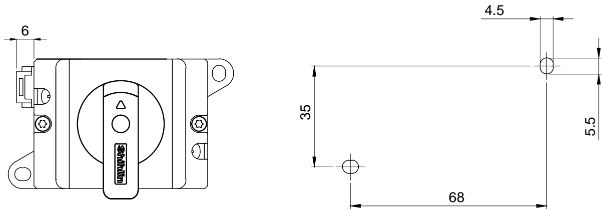
安裝孔尺寸
